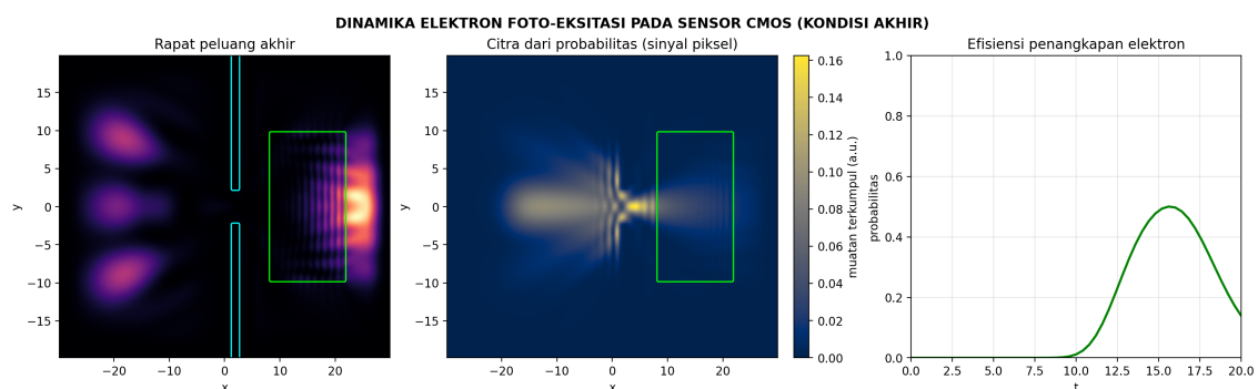
Gambar 7: Output program Kasus 7: fotodiode CMOS (rapat peluang, citra muatan terkumpul, dan efisiensi penangkapan)
